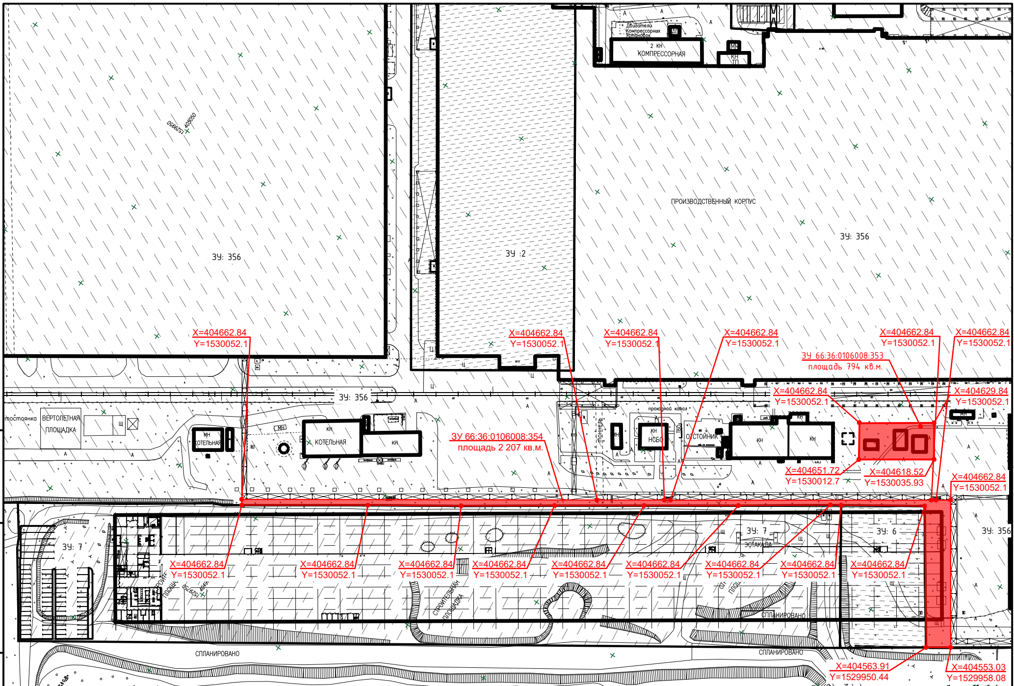
Схема планировочной организации земельного участка
